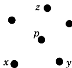
Fig. 7. \text{int}(S/xy) \neq \text{int}(S/x) \cap \text{int}(S/y) .
